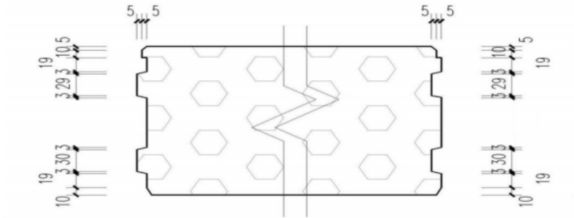
图 3 外墙板双凹凸型槽口构造示意图
